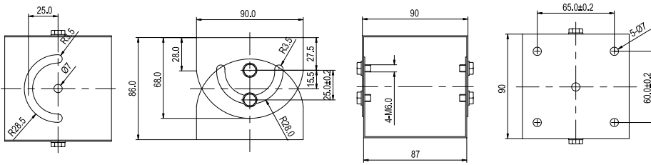
万向节支架尺寸
